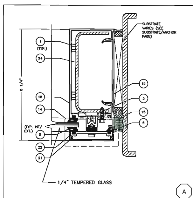
JAMB
