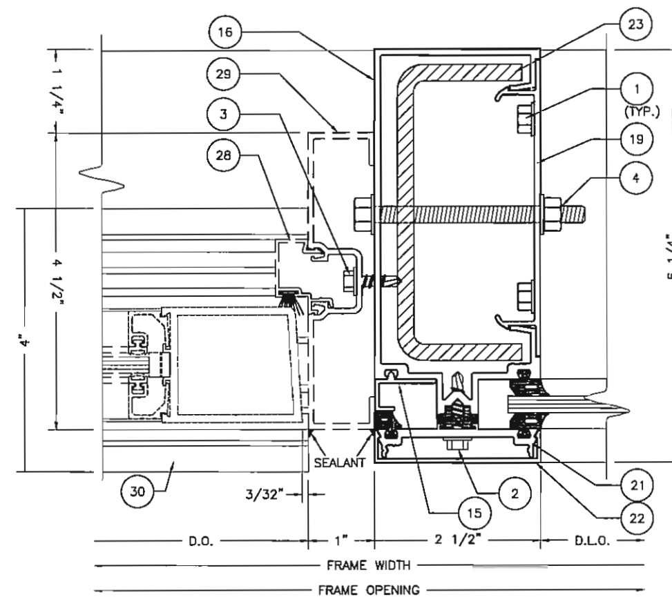
11 7 DETAIL SCALE: 1/2" = 1'-0"
