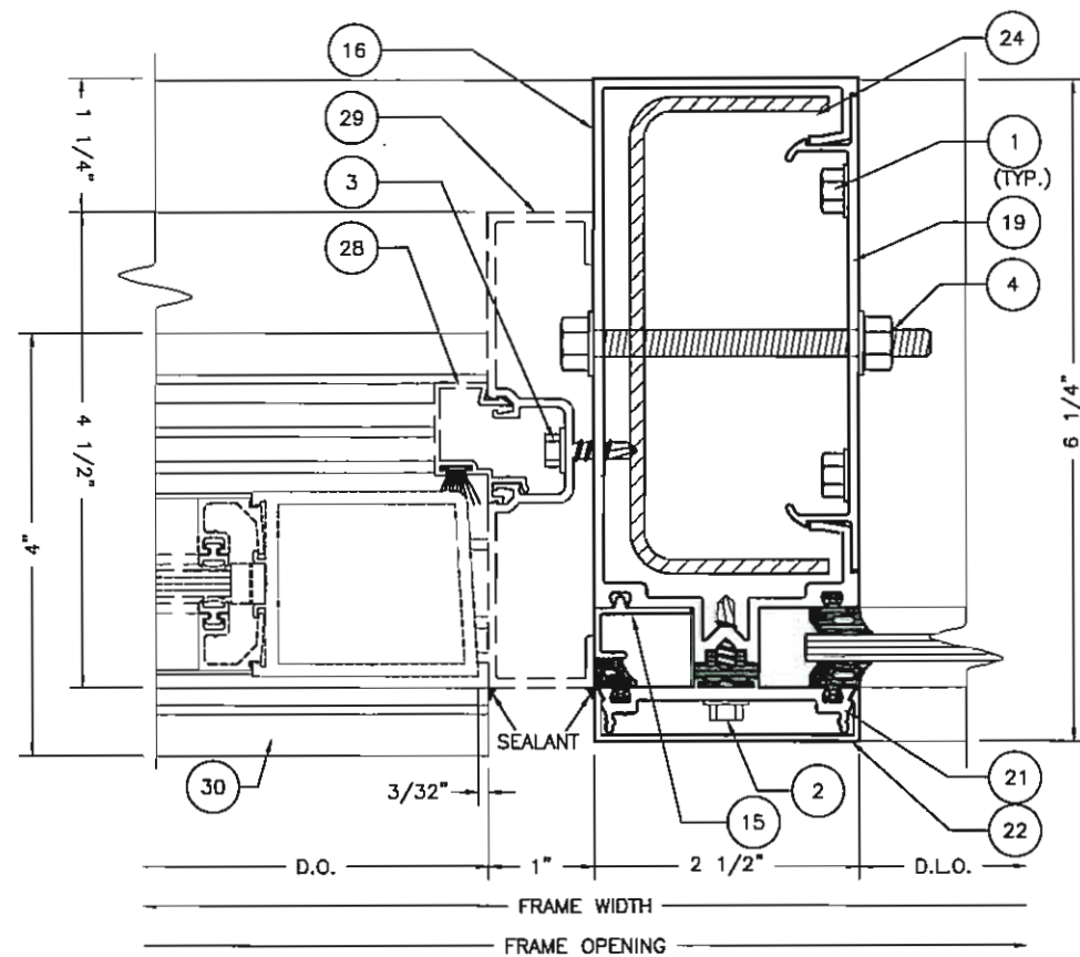
10 DETAIL 7 SCALE: 1:2
