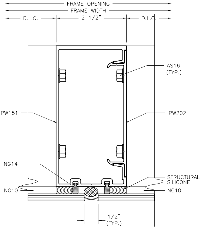
B.G. MULLION 1:2
