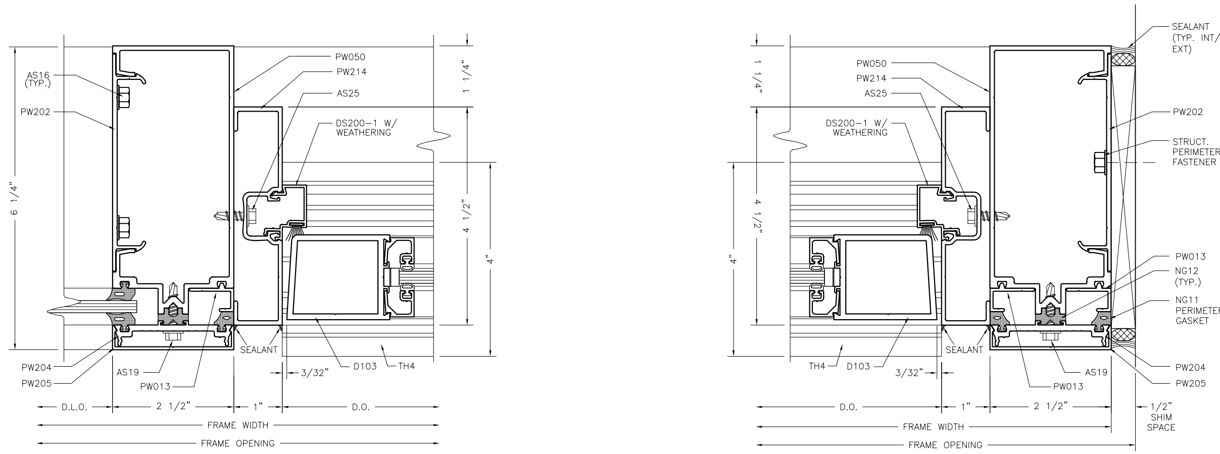
INT. DOOR JAMB 1:2
