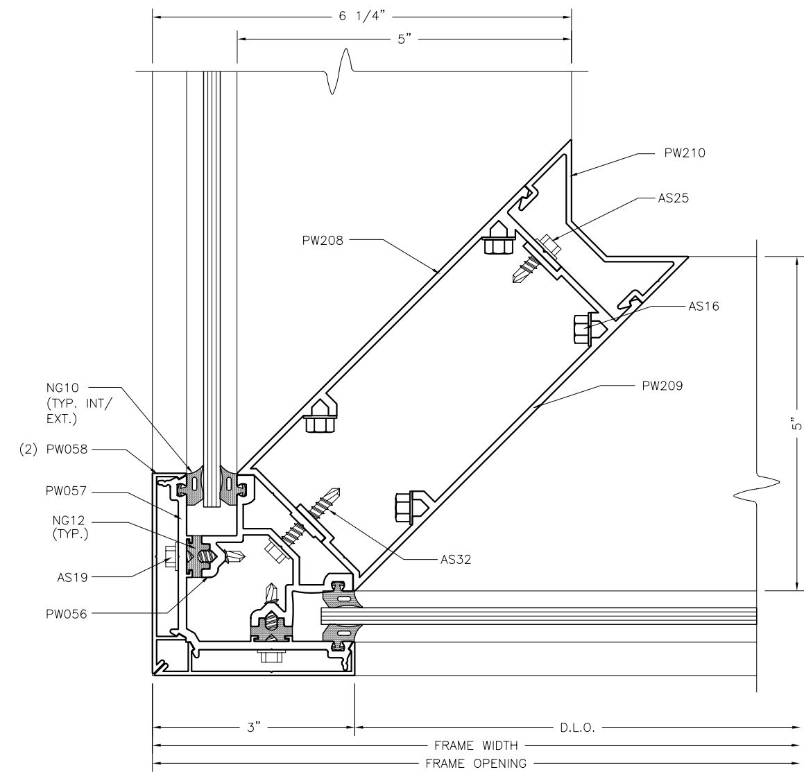
90° CORNER 1:2
