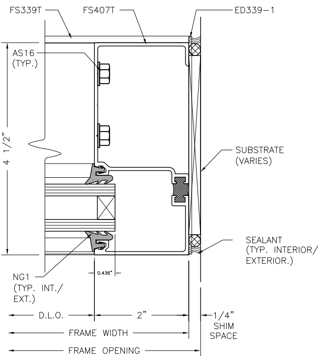
JAMB 1:2
