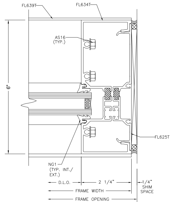
STANDARD JAMB
