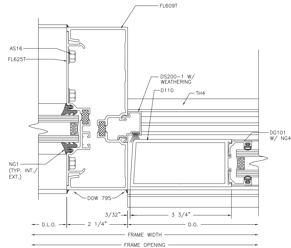
DOOR SIDELITE
