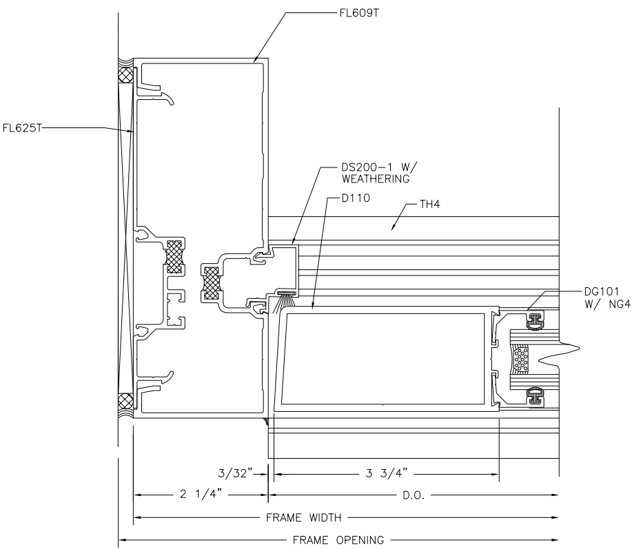
DOOR JAMB
