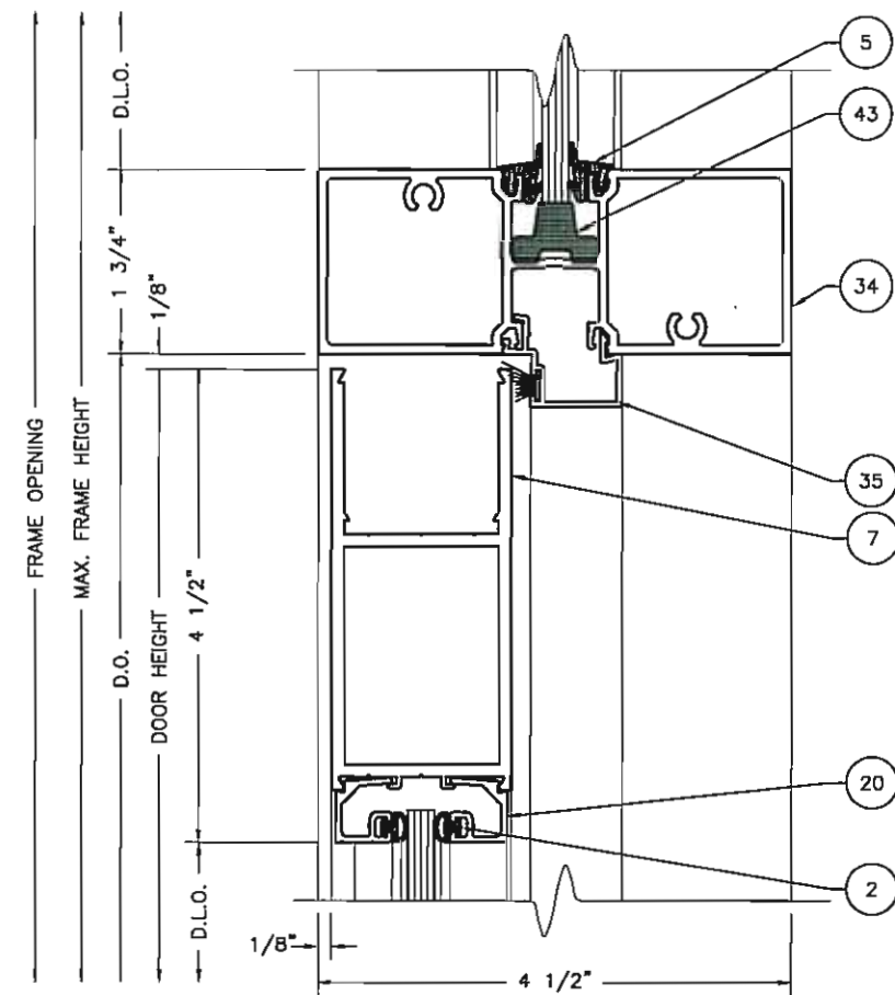
7 MS & WS INT DOOR HEADER 8 SCALE: 1:2
