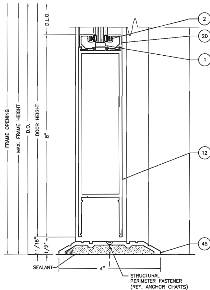
6 MS & WS THRESHOLD 8 SCALE: 1:2
