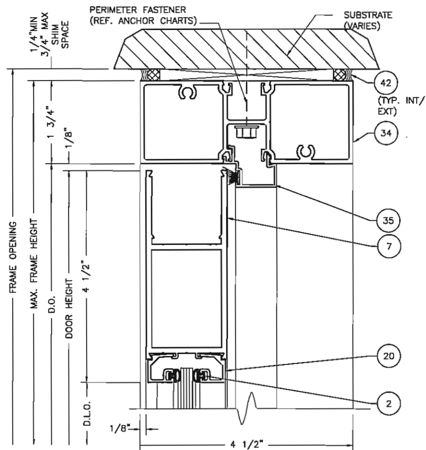
5 MS & WS DOOR HEADER 9 SCALE: 1:2
