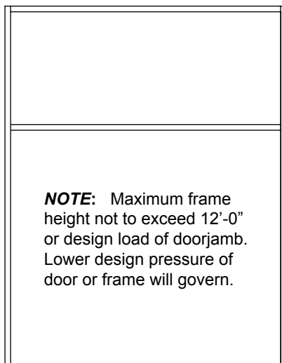
FRAME & TRANSOM
