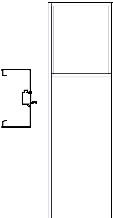
FRAME & TRANSOM
