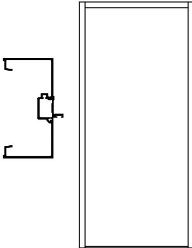
FRAME & TRANSOM
