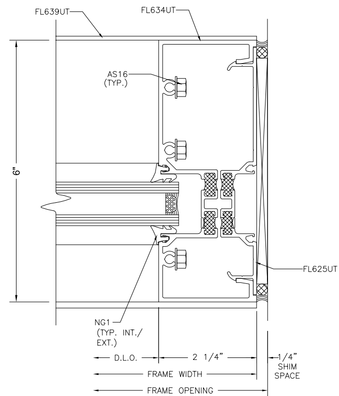
STANDARD JAMB
