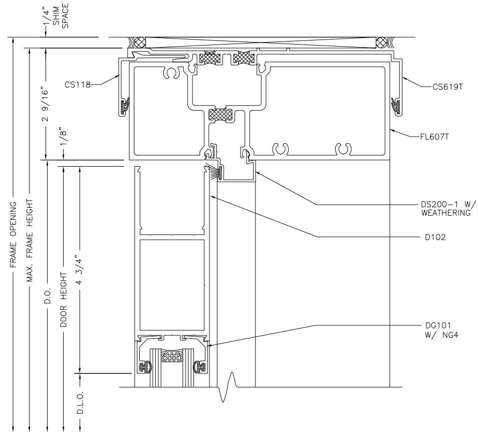
DOOR HEAD
