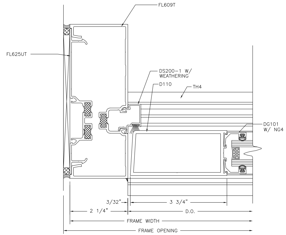
DOOR JAMB
