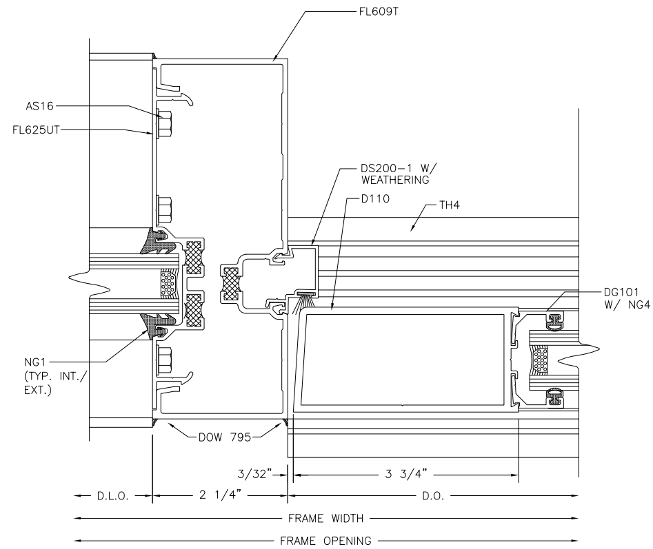
DOOR SIDELITE
