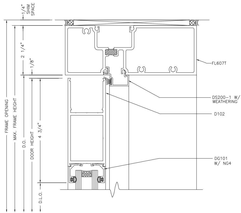
DOOR HEAD
