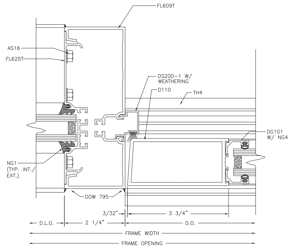
DOOR SIDELITE
